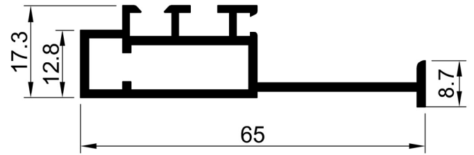
50 E 54 Ağırlık: 0,712 kg/m
