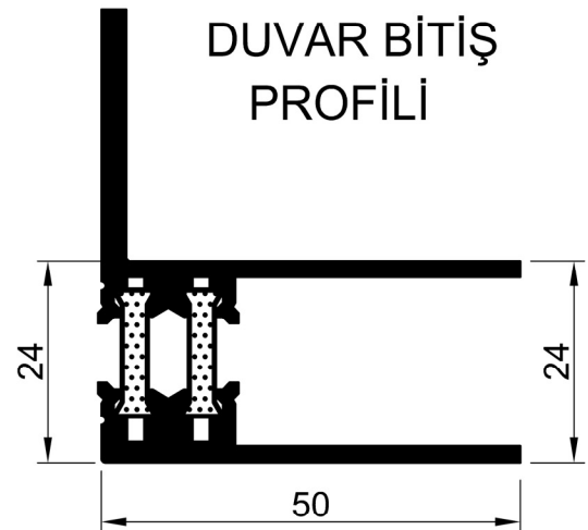
50 E 95 Ağırlık: 1,224 kg/m
