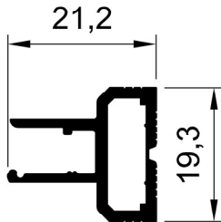
2742 Ağırlık: 0,269 kg/m
