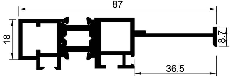
50 E 159 1.174 kg/m
