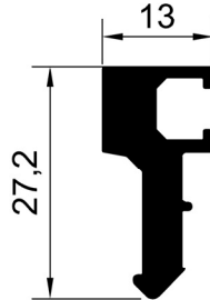
50 E 160 Ağırlık: 0,452 kg/m
