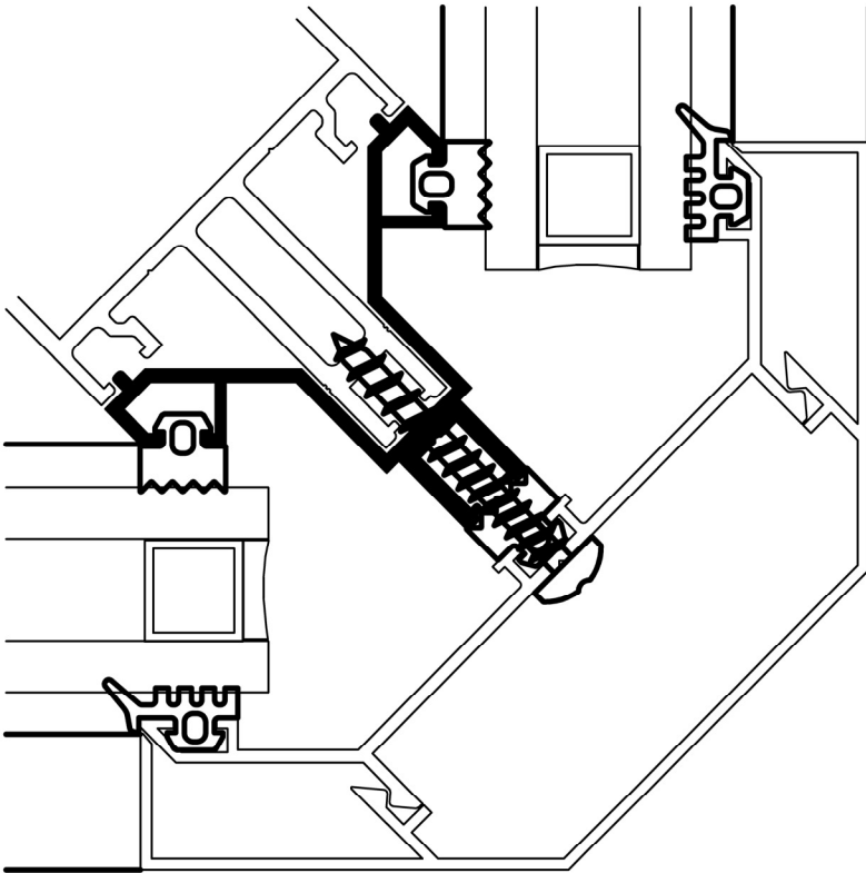
50 E 51 Ağırlık: 0,634 kg/m
