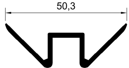
50 E 125 Ağırlık: 0,414 kg/m
