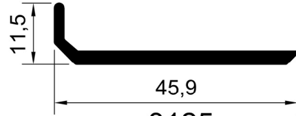
3125 Ağırlık: 0,335 kg/m
