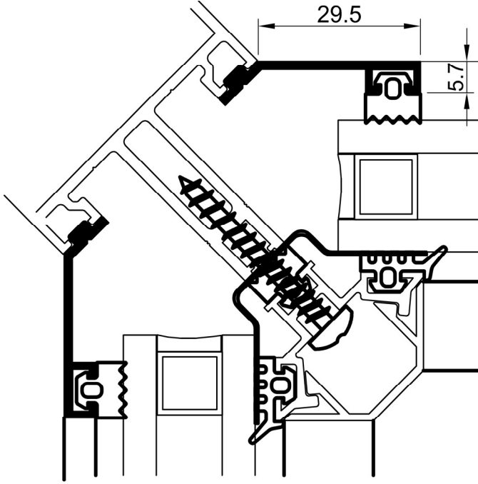
50 E 52 Ağırlık: 0,219 kg/m
