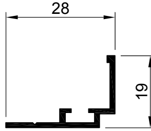
40 E 87 AĞIRLIK : 0.195 kg/m
