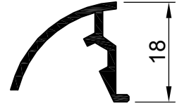
40 E 86 AĞIRLIK : 0.180 kg/m
