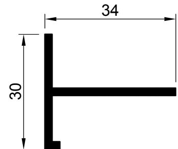
92-447 AĞIRLIK : 0.346 kg/m
