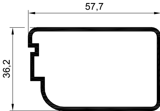
50 E 87 AĞIRLIK : 0.768 kg/m JX: 5.82 cm 4 JY: 12.15 cm 4
