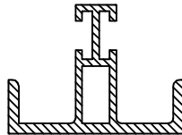
40 D 12 TOZ TUTUCU PLASTİĞİ (3 mt)
