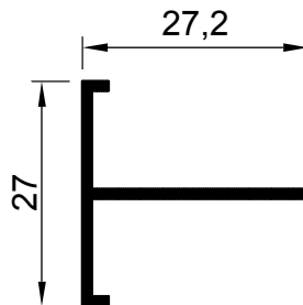
00-1322 AĞIRLIK : 0.185 kg/m
