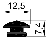
05-2306 AĞIRLIK : 0.160 kg/m
